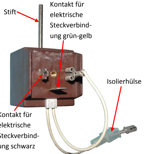
Isolierhülle
